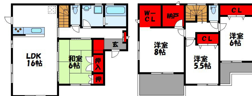
【間取り図】
